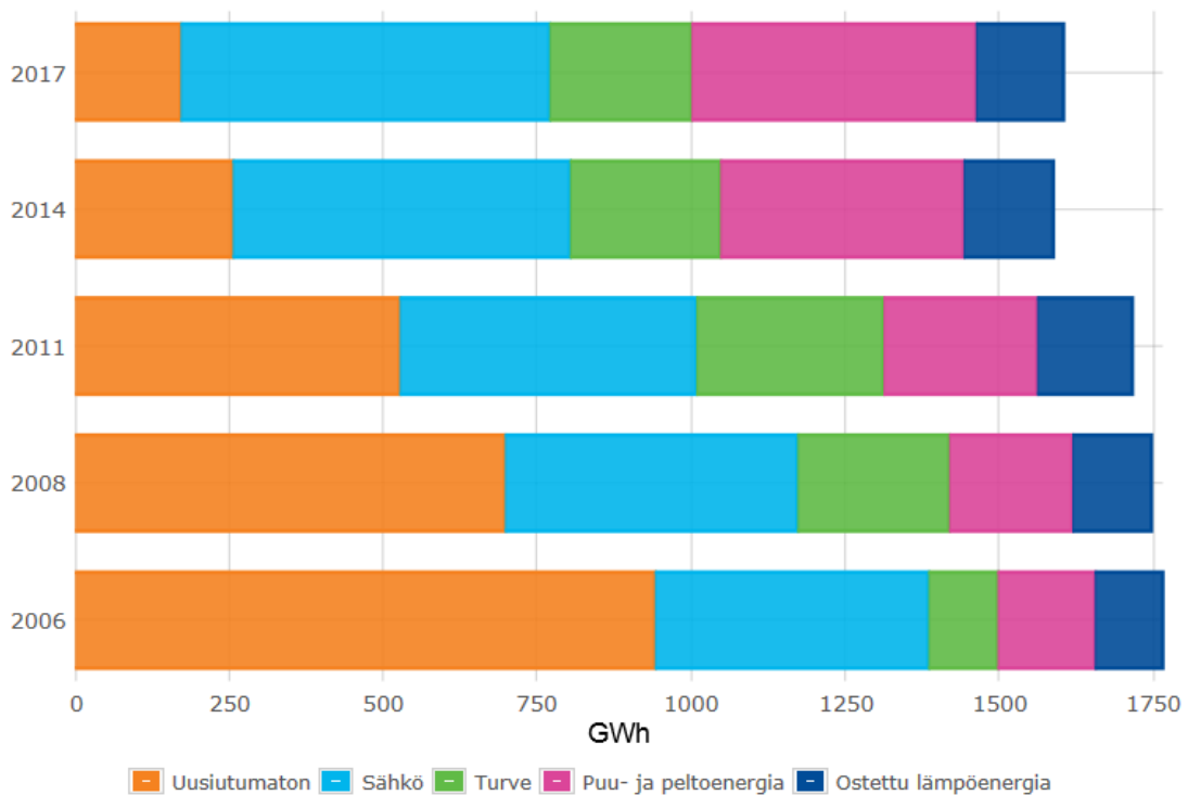
Kuva 5 Kasvihuoneyritysten energiankulutus 2006-2017. Uusiutumaton energia kuvaa tässä fossiilista energiaa. Sähköenergiaa ei ole laskettu primaarienergiana.
