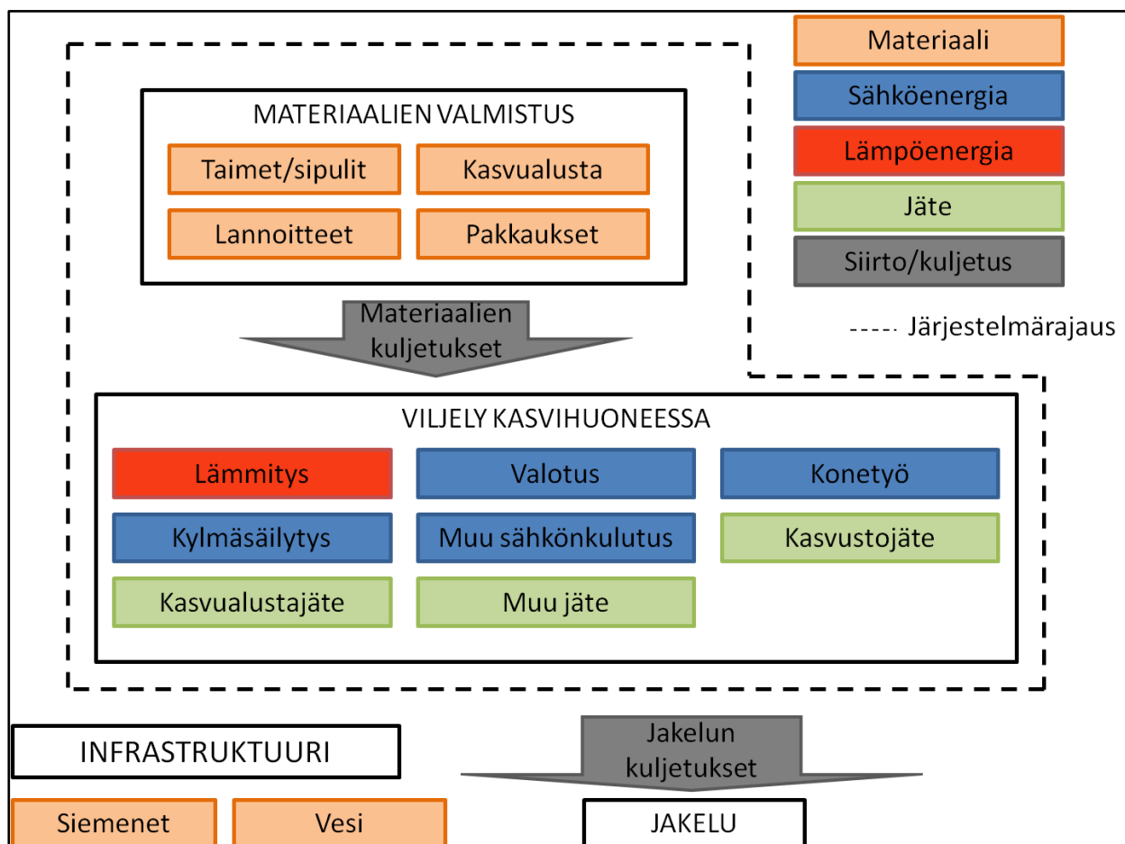
Kuva 1. Kasvihuoneviljelyn energia- ja materiaalivirrat sekä järjestelmärajaukset.
